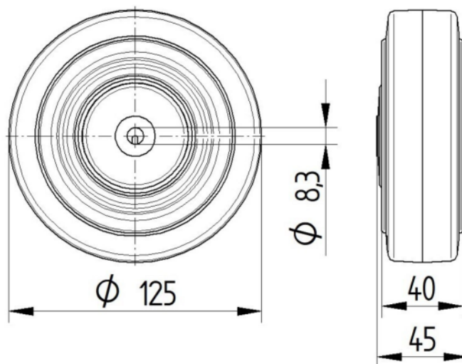
XLP125x40-Ø8,3 NL45
